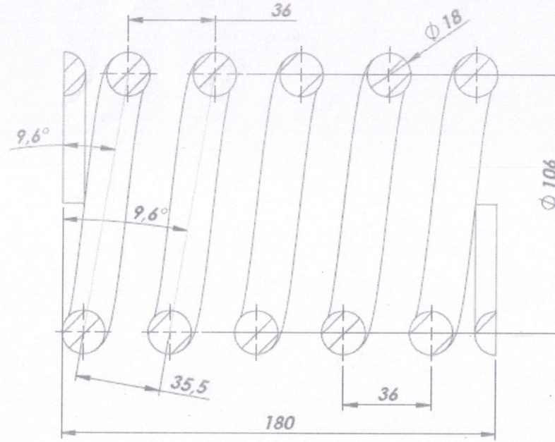
KESİT A-A
